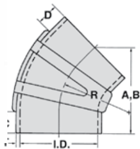
45° Elbow
